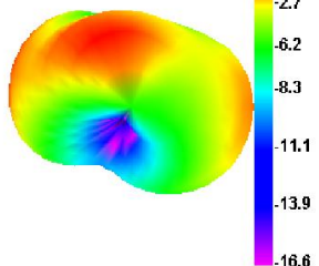
860.000MHz
