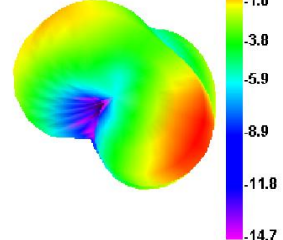
920.000MHz
