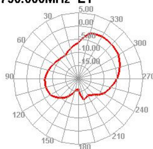
750.000MHz E1
