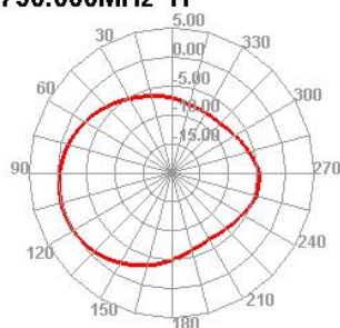
750.000MHz H
