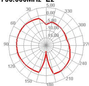
750.000MHz E2
