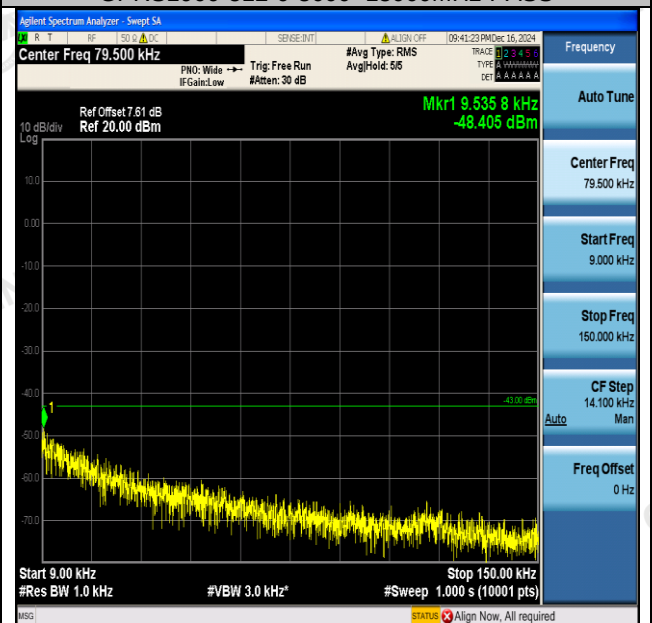
GPRS1900-661-0-0.009~0.15MHz-PASS
