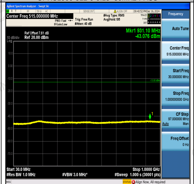
GPRS1900-512-0-30-1000MHz-PASS
