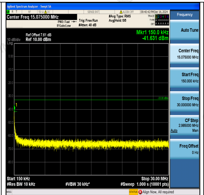
GPRS1900-512-0-0.15-30MHz-PASS
