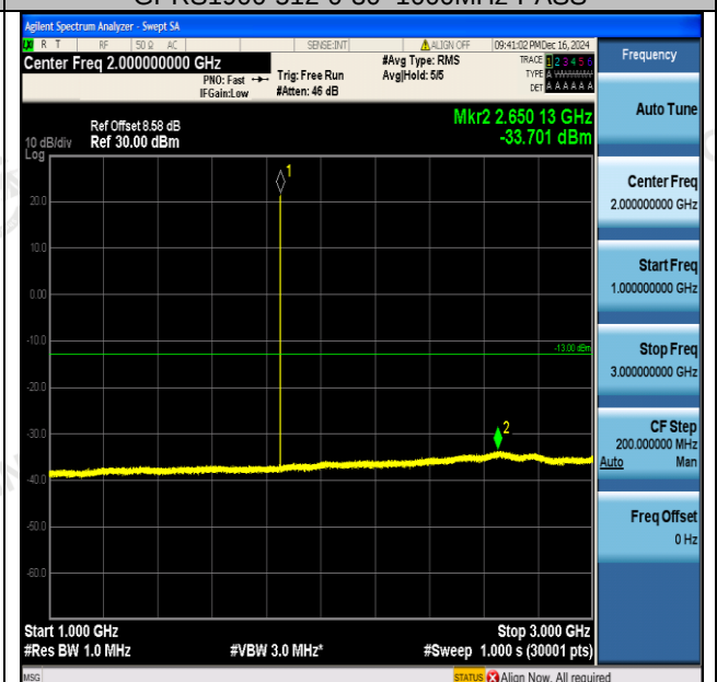
GPRS1900-512-0-1000-3000MHz-PASS
