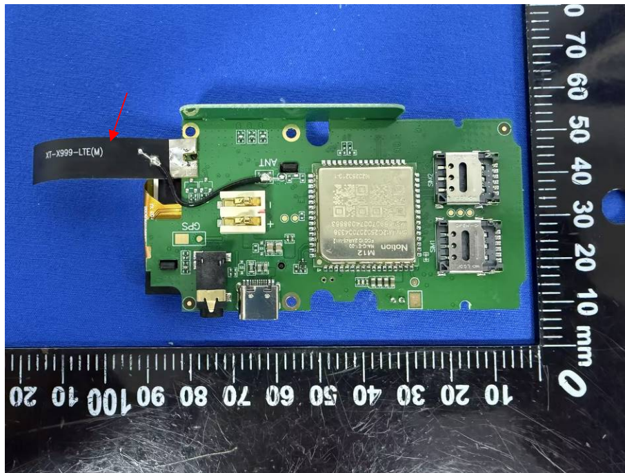
LTE Antenna
