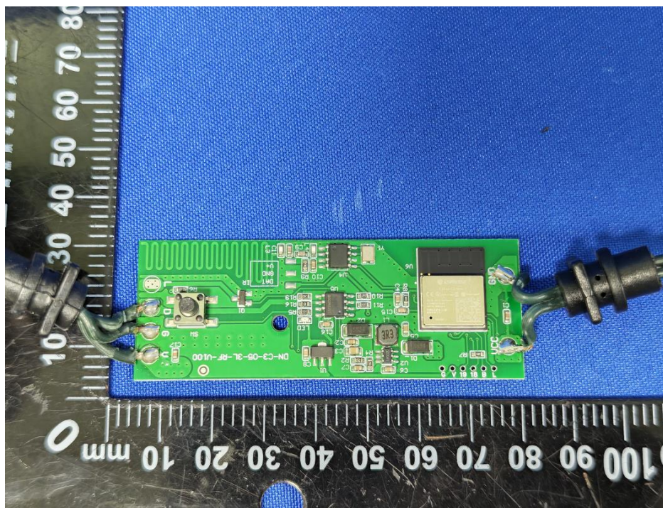
BT ANT
