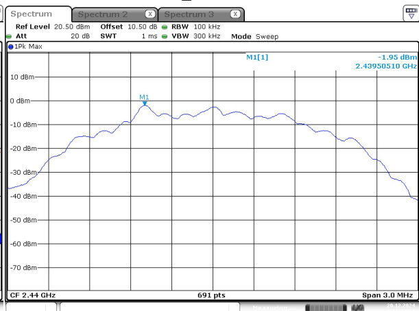
2M_Middle -1
