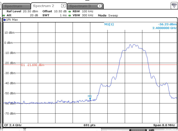
3EDR_Low -2
