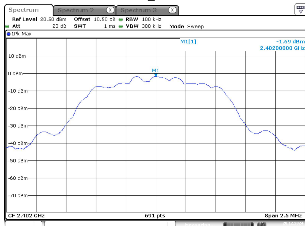
3EDR_Low -1
