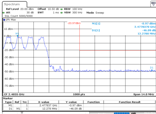
DH1_Hopping_Upper
