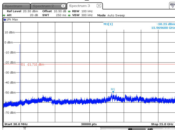
2EDR_Low -3
