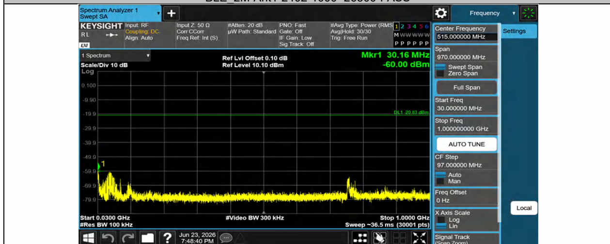
BLE_2M-Ant1-2440-30~1000-PASS
