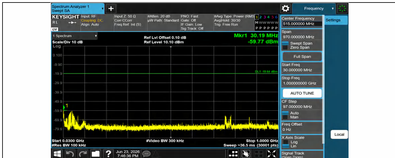
BLE_2M-Ant1-2402-30~1000-PASS
