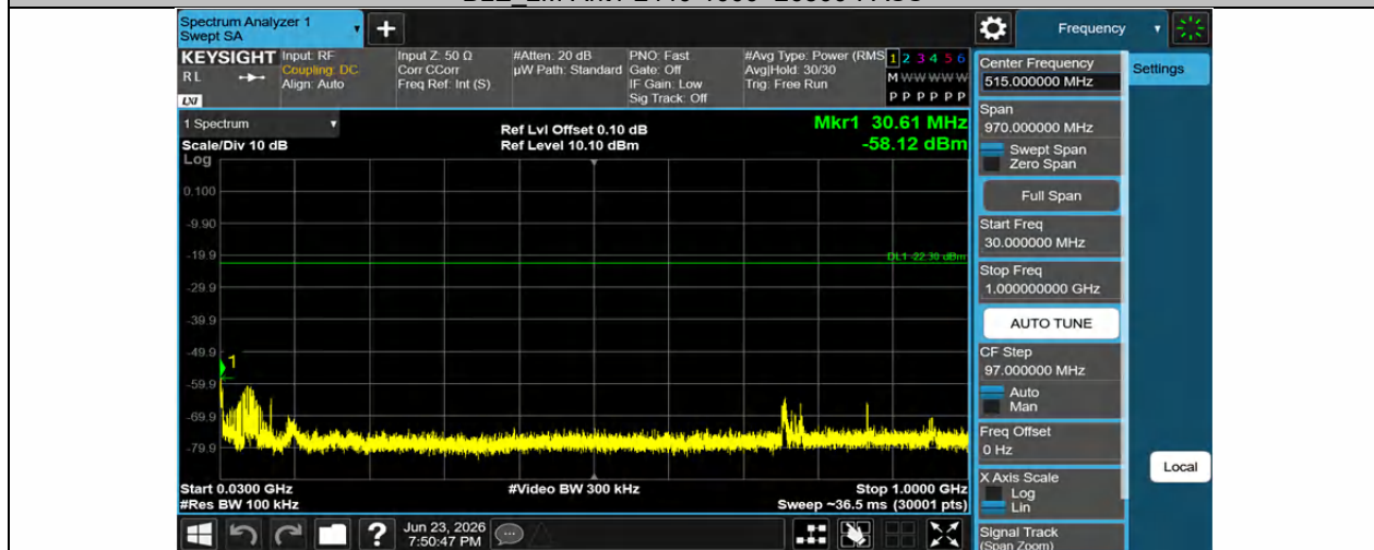
BLE_2M-Ant1-2480-30~1000-PASS
