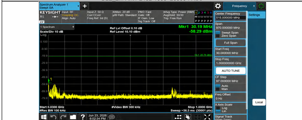
BLE_2M-Ant1-2440-30~1000-PASS
