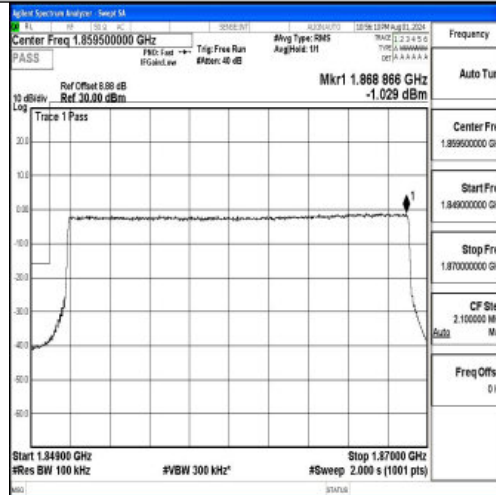
Band2-20MHz-QPSK-18700-100RB#0-PASS
