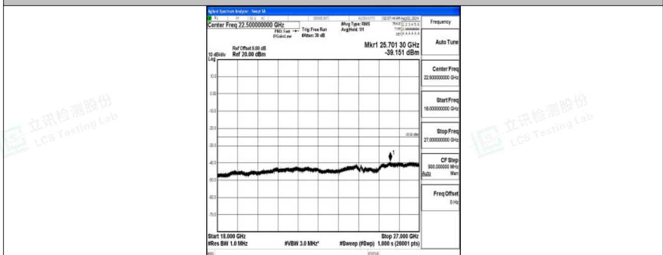
Band7-15MHz-16QAM-20825-1RB#0-18000~27000-PASS
