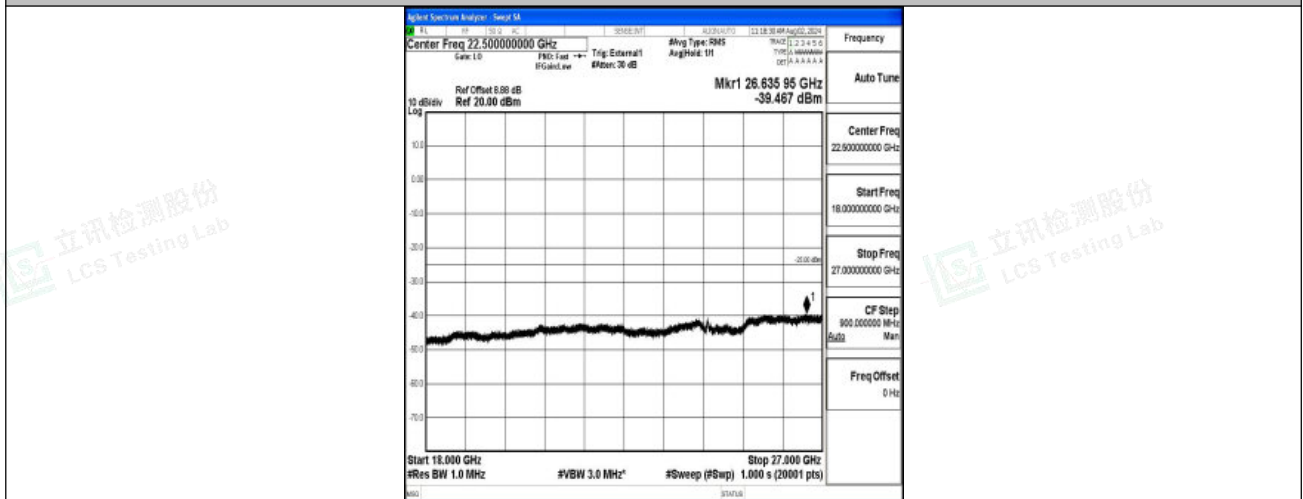
Band38-15MHz-QPSK-38000-1RB#0-18000~27000-PASS
