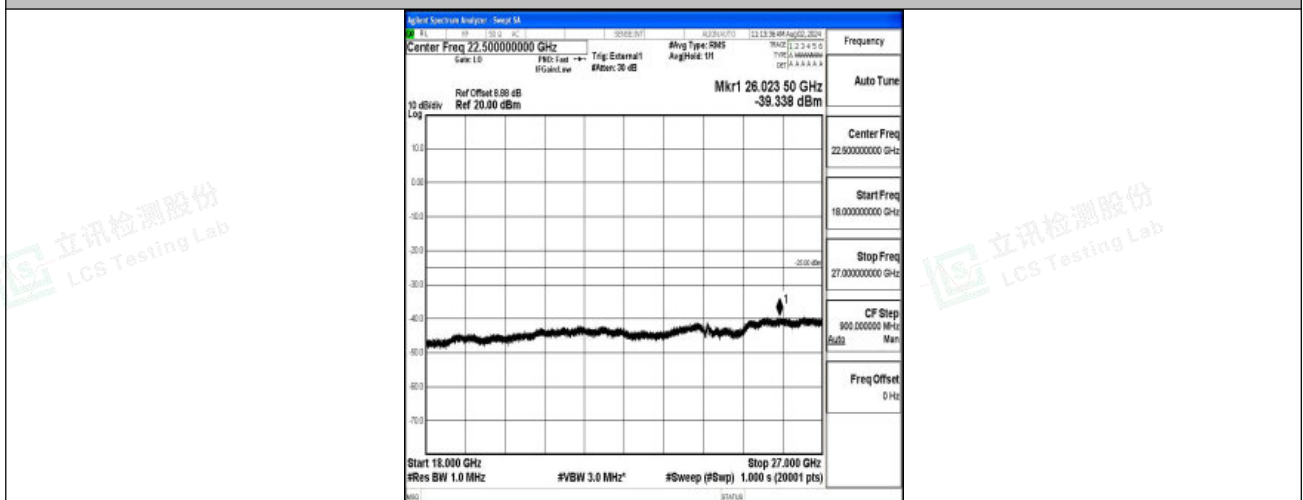
Band38-15MHz-QPSK-37825-1RB#0-18000~27000-PASS
