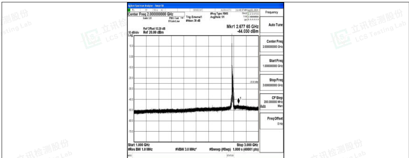
Band38-20MHz-QPSK-37850-1RB#0-1000~3000-PASS
