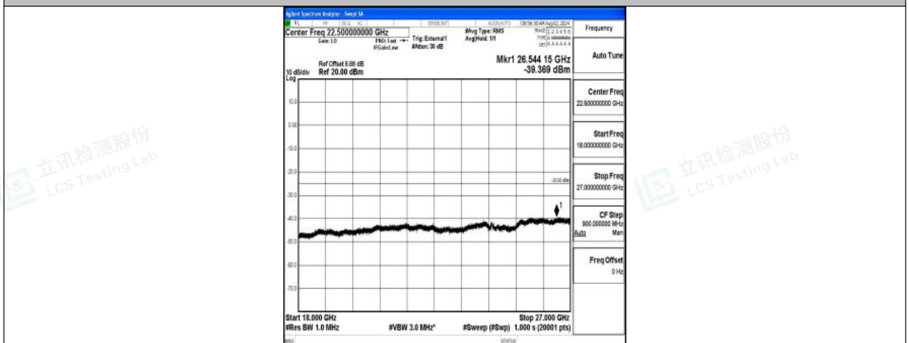
Band41-20MHz-QPSK-41490-1RB#0-18000~27000-PASS
