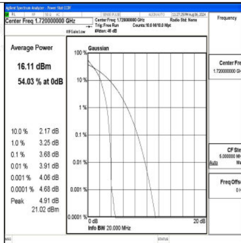
Band66-20MHz-QPSK-132072-1RB#0-PASS
