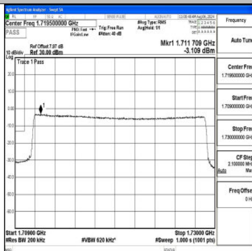
Band66 20MHz QPSK 132072 100RB#0
