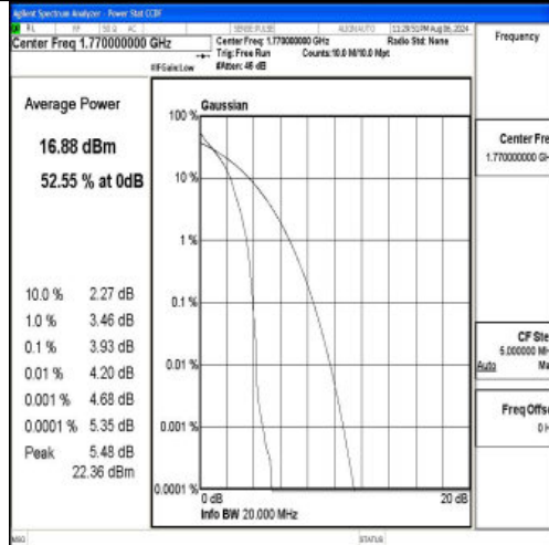
Band66-20MHz-QPSK-132572-1RB#0-PASS
