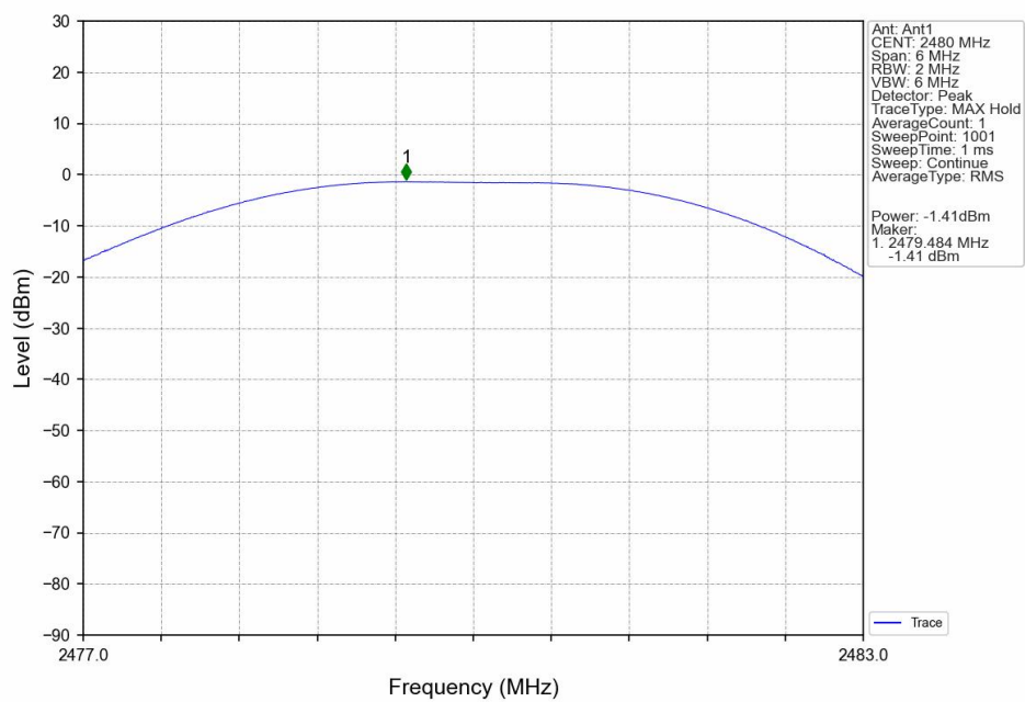
Peak Power NVNT BLE 2M 2480MHz Ant1
