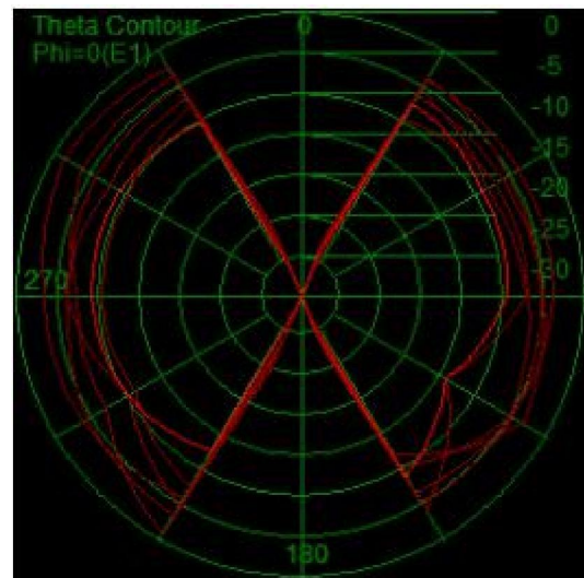
Passive -Freq2420.00MHz
