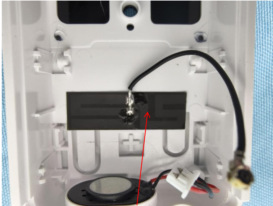
BLE&WLAN ANT
