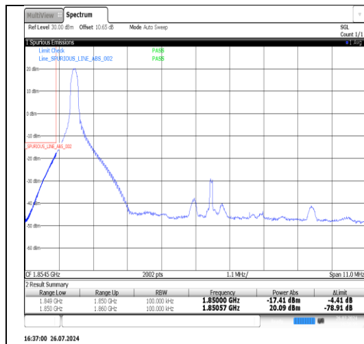
Band2-10MHz-QPSK-18650-1RB#49-PASS
