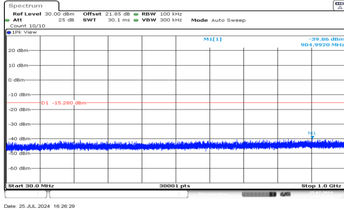
DH5_Ant1_2480_30-1000
