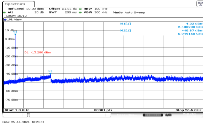
DH5_Ant1_2480_1000-26500
