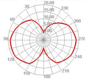
LTE71 133422 TRP Phi=45
