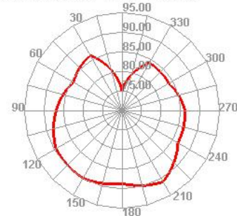
LTE7 3400 TIS Phi=45
