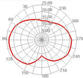
LTE5 20600 TRP Phi=45
