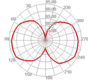
LTE71 68886 TIS Phi=45
