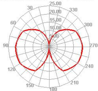
LTE28 27435 TRP Phi=45
