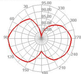
LTE12 5130 TIS Phi=45
