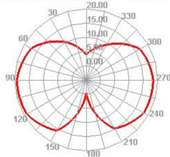
LTE28 27610 TRP Phi=45
