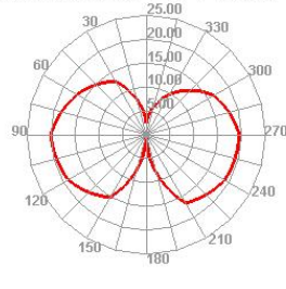
LTE12 23130 TRP Phi=45
