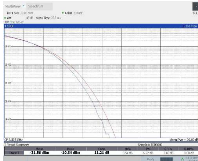
Band7-10MHz-QPSK-20800-50RB#0
