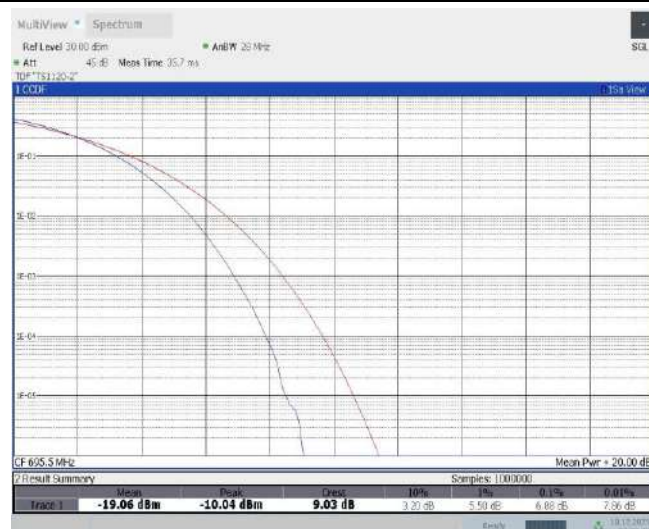
Band71-5MHz-QPSK-133447-25RB#0
