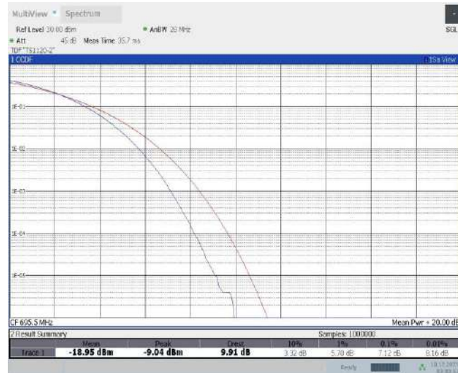
Band71-10MHz-QPSK-133172-1RB#0
