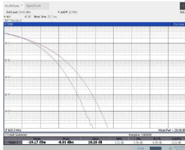
Band71-5MHz-QPSK-133147-25RB#0
