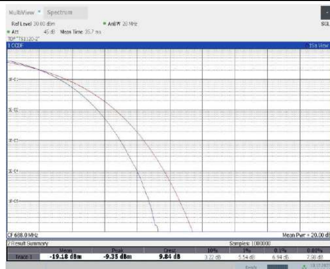
Band71-20MHz-QPSK-133372-100RB#0
