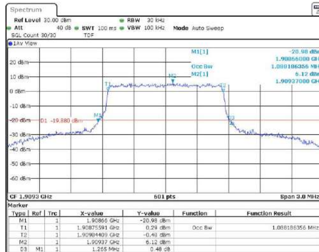
Band2-3MHz-QPSK-18615-15RB#0
