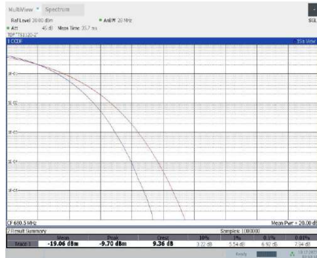
Band71-5MHz-QPSK-133297-25RB#0
