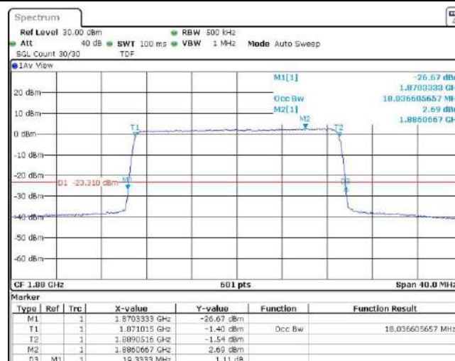
Band2-20MHz-16QAM-18900-100RB#0
