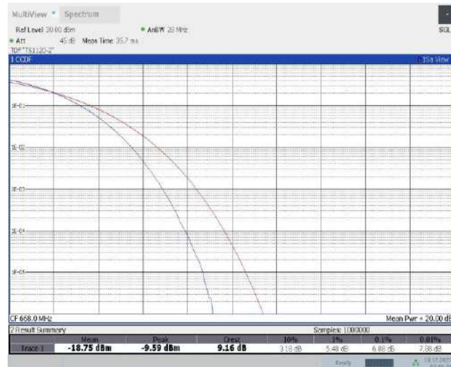
Band71-10MHz-QPSK-133172-50RB#0
