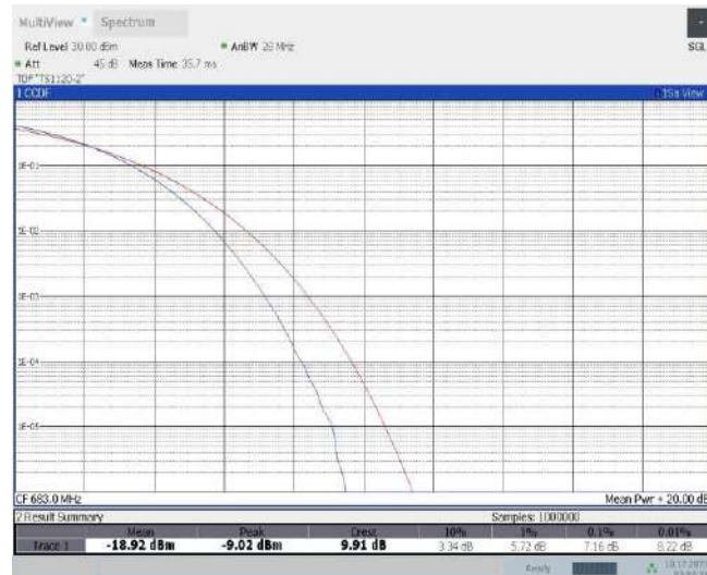
Band71-20MHz-16QAM-133372-1RB#0
