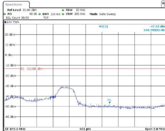
Band5-3MHz-QPSK-20635-1RB#14
