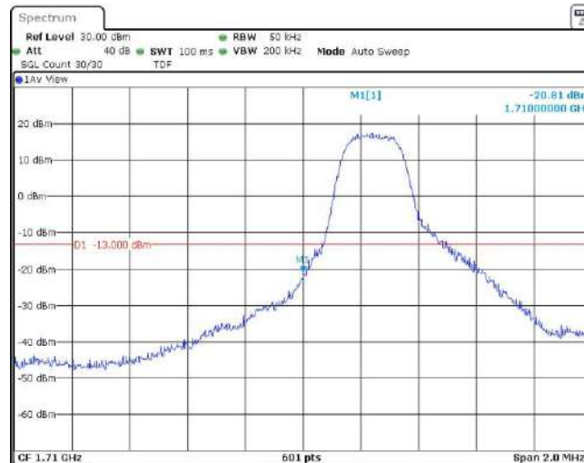
Band4-3MHz-QPSK-19965-1RB#14
