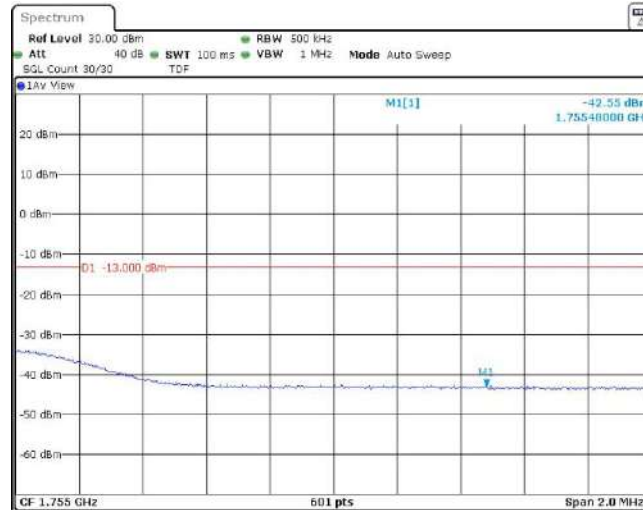
Band4-20MHz-QPSK-20300-1RB#99
