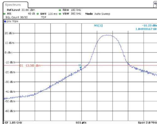
Band2-5MHz-QPSK-18625-1RB#24
