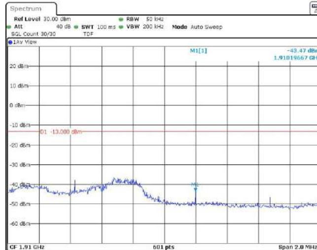
Band2-3MHz-QPSK-19185-1RB#14
