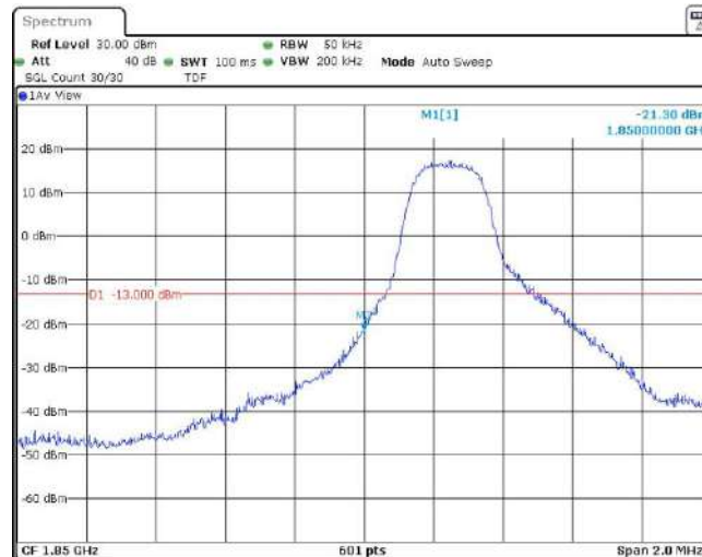
Band2-3MHz-QPSK-18615-1RB#14
