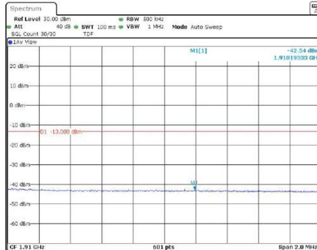
Band2-20MHz-QPSK-19100-1RB#99
