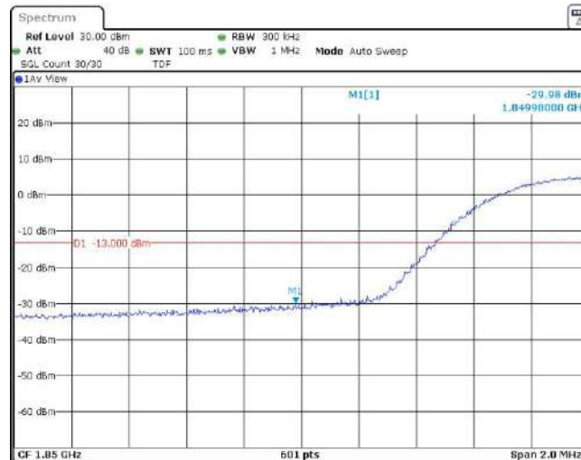
Band2-15MHz-QPSK-18675-1RB#74
