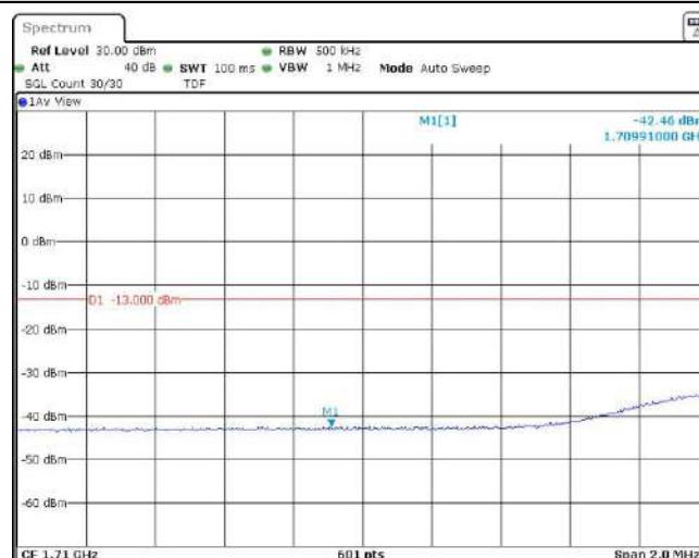
Band4-20MHz-QPSK-20050-100RB#0
