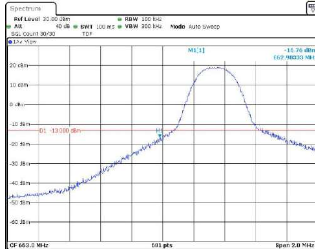
Band71-5MHz-QPSK-133147-1RB#24
