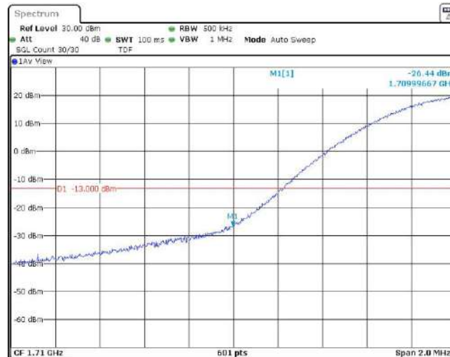
Band66-20MHz-16QAM-132072-1RB#99
