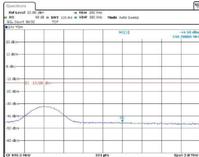
Band71-10MHz-QPSK-133422-1RB#49
