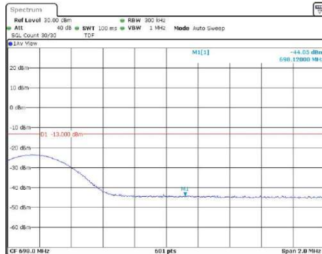
Band71-15MHz-QPSK-133397-1RB#74
