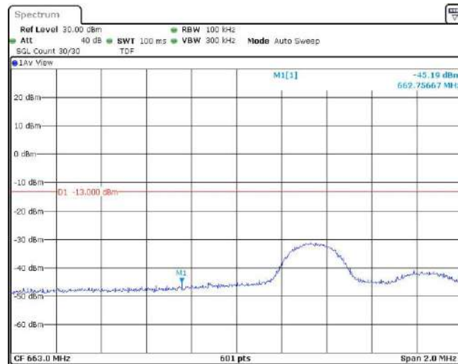
Band71-5MHz-QPSK-133147-25RB#0
