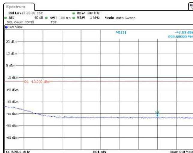
Band71-20MHz-16QAM-133372-1RB#99
