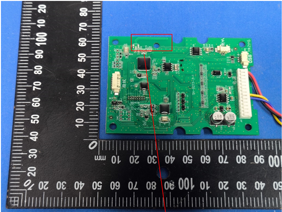
LE Antenna
