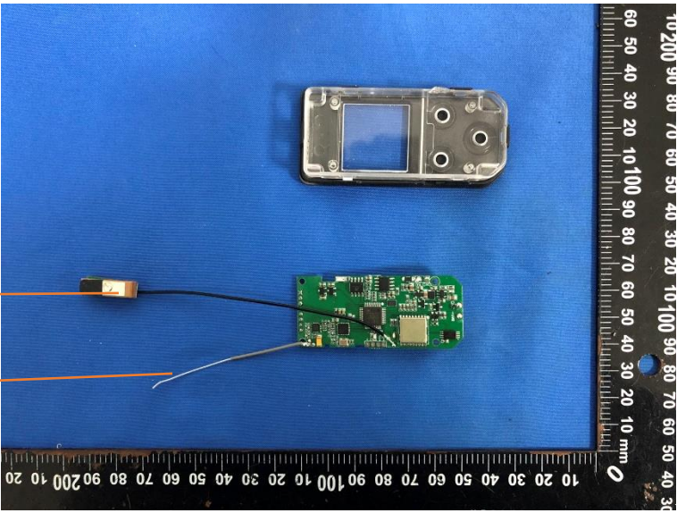
2.4G antenna
