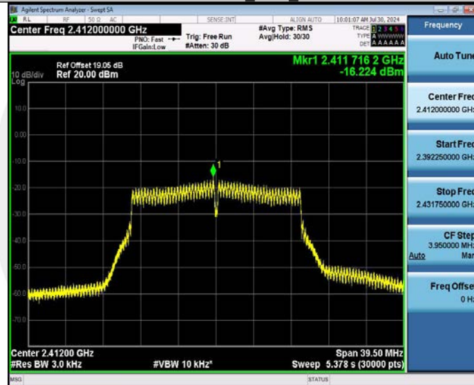
11N20MIMO_Ant2_2412
