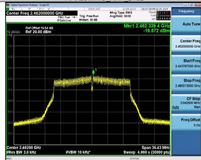
11AX20MIMO_Ant2_2462
