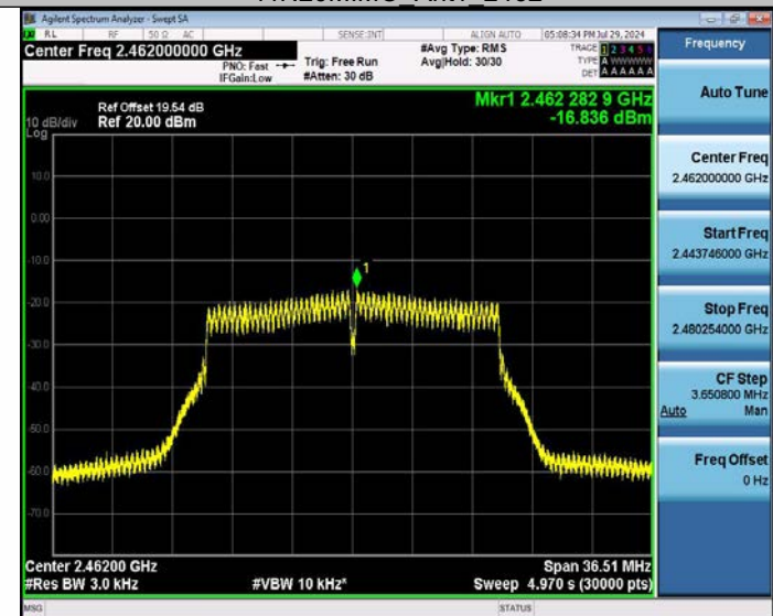
11N20MIMO Ant2 2462
