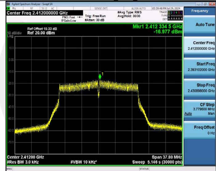
11AX20MIMO_Ant2_2412
