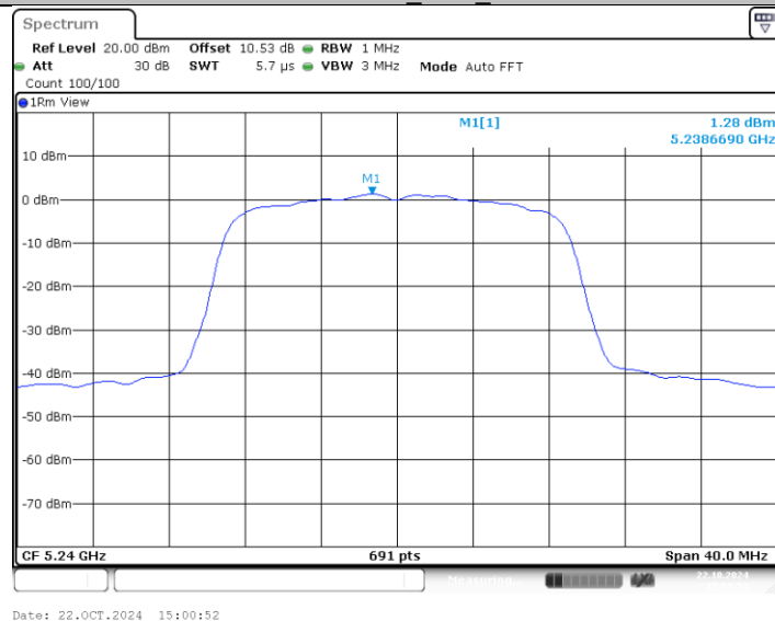
11AX20MIMO_Ant2_5240
