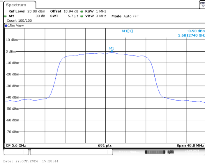
11AX20MIMO_Ant2_5600
