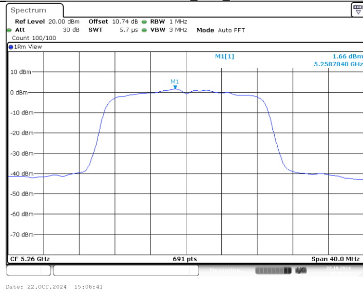
11AX20MIMO_Ant2_5260
