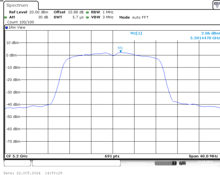
11AX20MIMO_Ant2_5200
