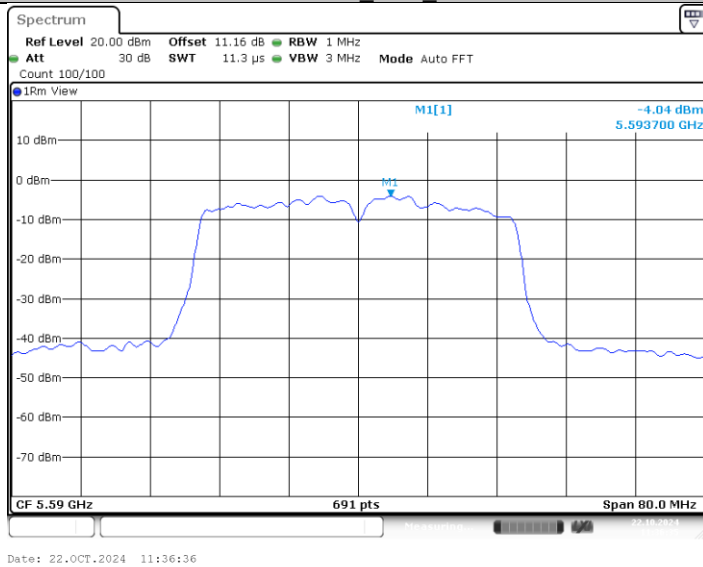
11N40MIMO_Ant2_5590
