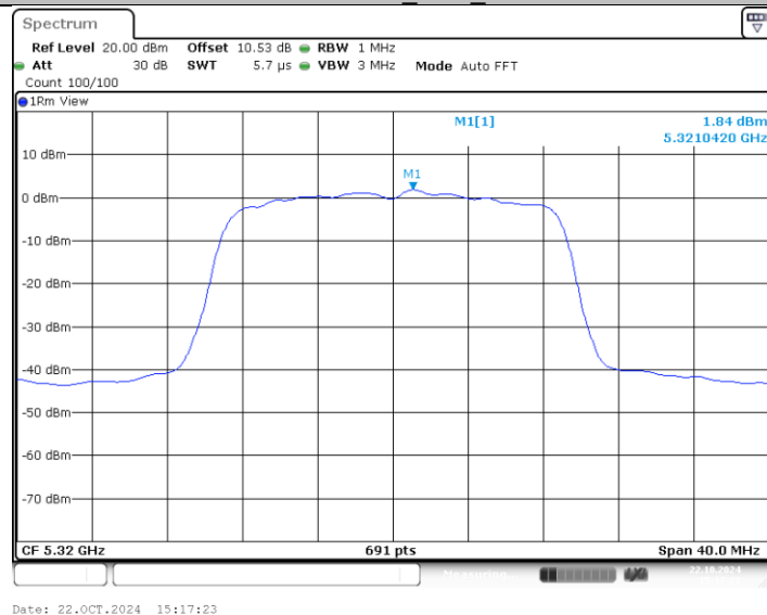
11AX20MIMO_Ant2_5320
