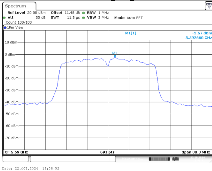
11AC40MIMO_Ant2_5590
