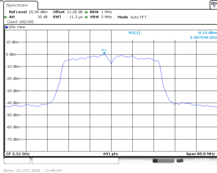
11AC40MIMO_Ant2_5310
