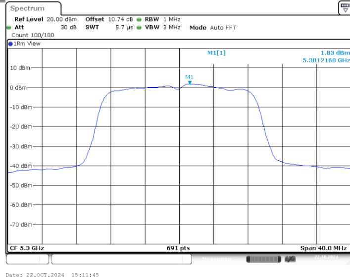
11AX20MIMO_Ant2_5300
