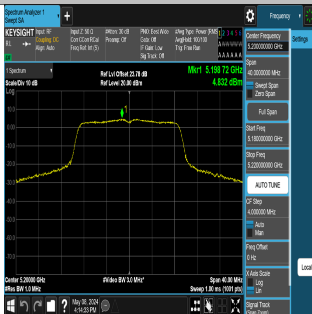
11N20MIMO-Ant1-5200-PASS
