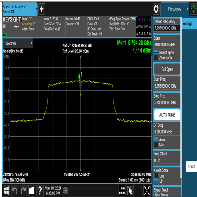
11N40MIMO-Ant1-5795-PASS
