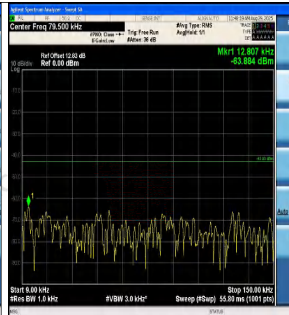
Band2-20MHz-QPSK-19100-100RB#0-0.009~0.15 -PASS
