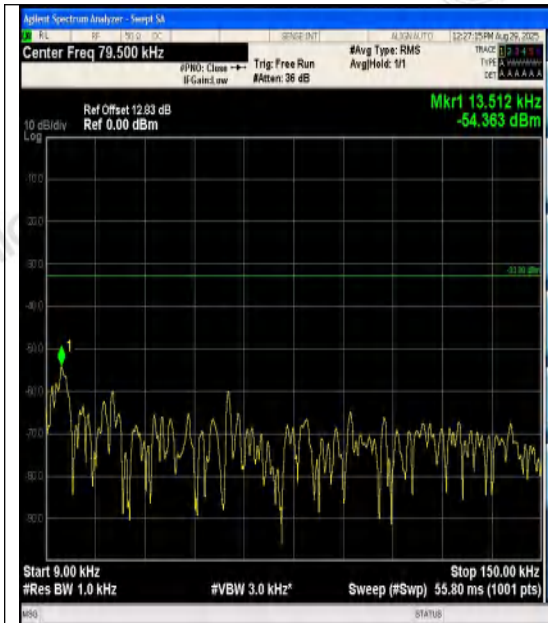
Band12-3MHz-QPSK-23025-15RB#0-0.009~0.15 -PASS
