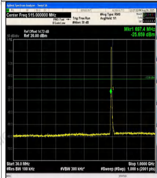
Band12-3MHz-QPSK-23025-15RB#0-30~1000-P ASS
