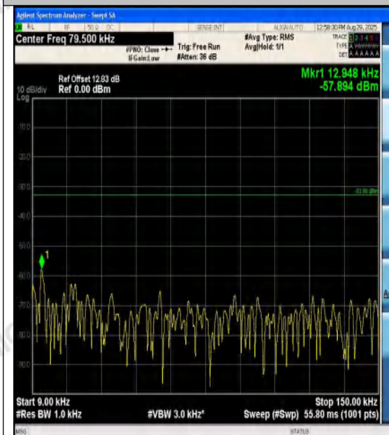
Band12-5MHz-QPSK-23155-25RB#0-0.009~0.15 -PASS
