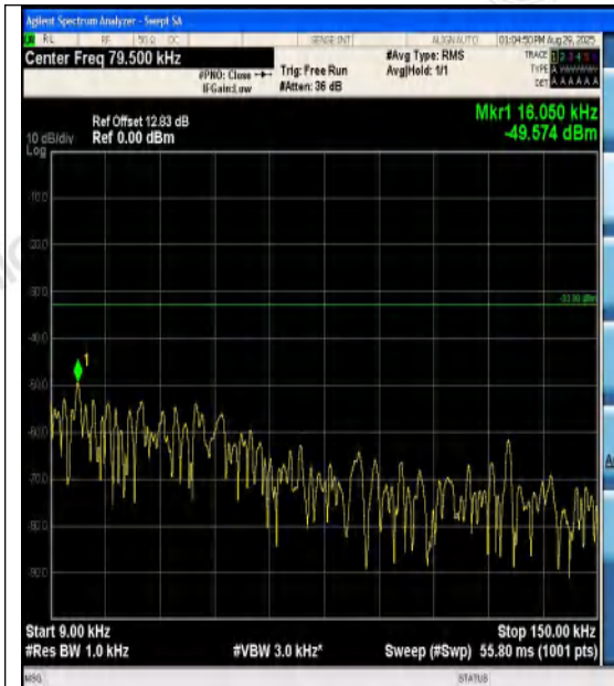
Band12-10MHz-QPSK-23095-1RB#0-0.009~0.15 -PASS
