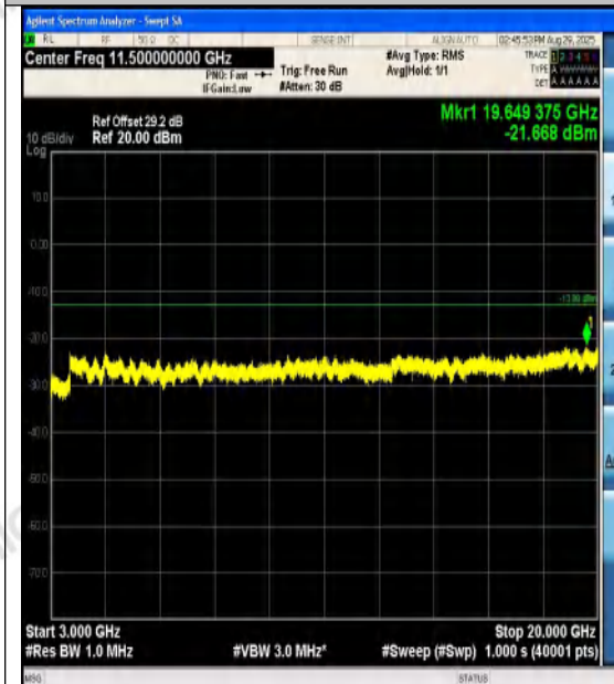
Band4-1.4MHz-QPSK-20393-1RB#0-3000~20000 -PASS
