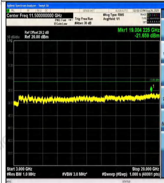
Band4-3MHz-QPSK-19965-15RB#0-3000~20000 -PASS
