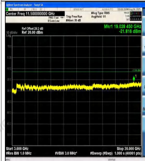
Band4-3MHz-QPSK-20385-1RB#14-3000~20000 -PASS
