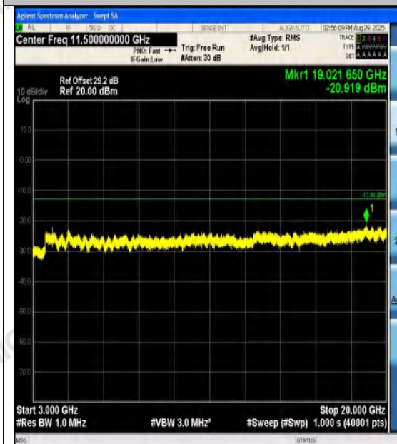
Band4-3MHz-QPSK-20175-1RB#14-3000~20000 -PASS
