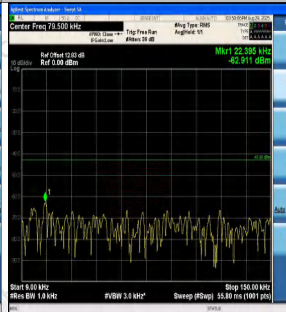
Band4-20MHz-QPSK-20050-100RB#0-0.009~0.15 -PASS
