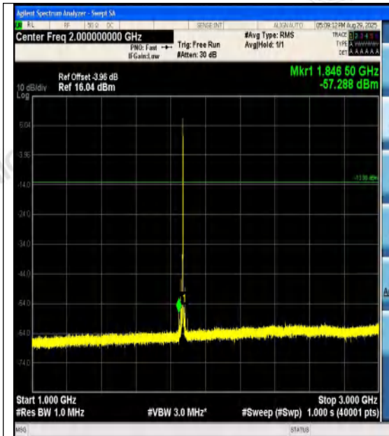
Band2-20MHz-QPSK-18700-1RB#99-1000~3000 -PASS
