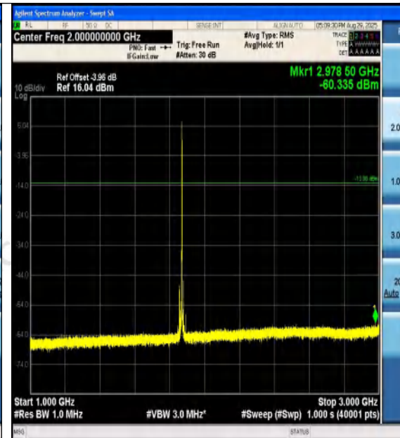
Band2-20MHz-16QAM-18700-1RB#99-1000~3000 -PASS
