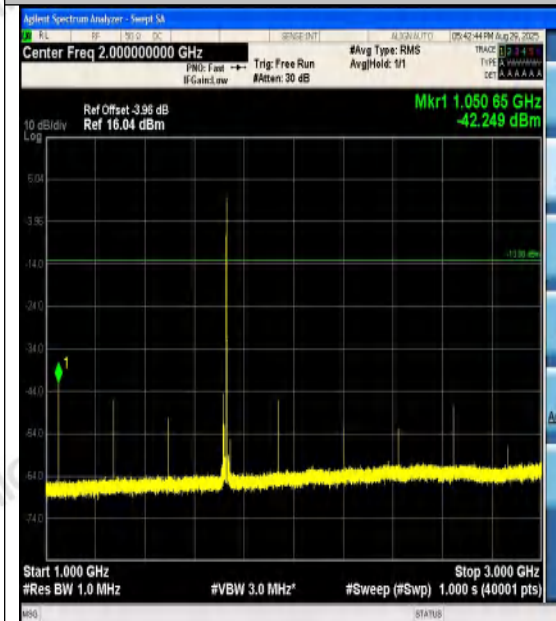
Band4-20MHz-QPSK-20050-1RB#99-1000~3000- -PASS
