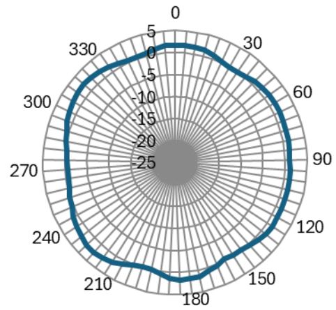
XY-2450MHz
