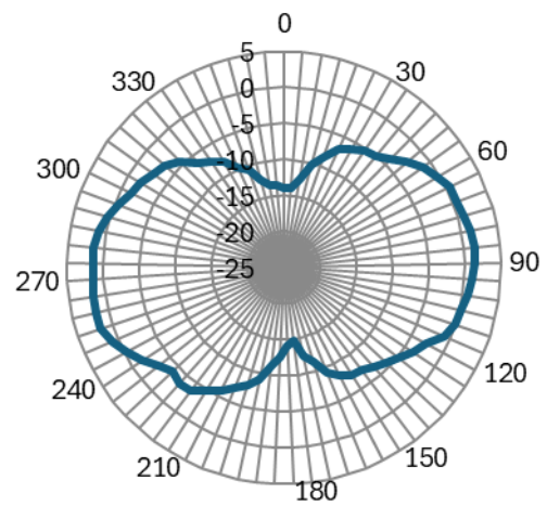
YZ-2450MHz
