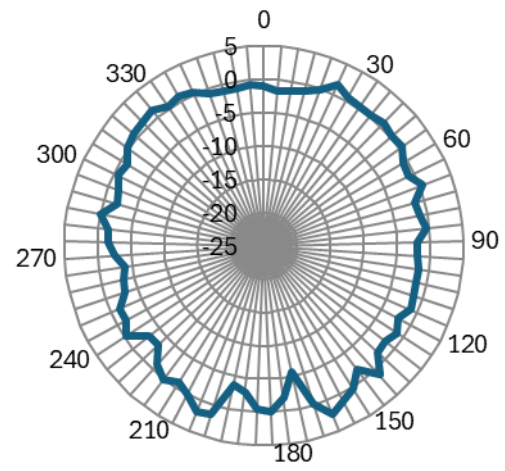
YZ-5450MHz
