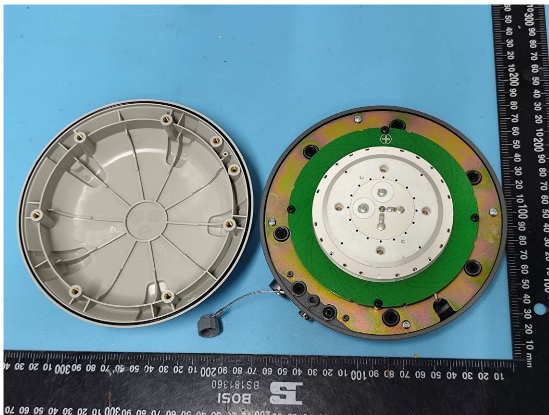
GSNSS antenna
