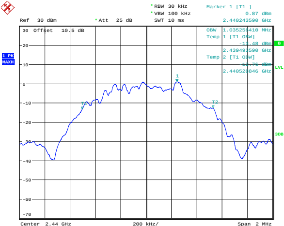
BLE 1Mbps_Middle_Channel
