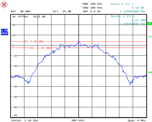
BLE 2Mbps_Middle_Channel
