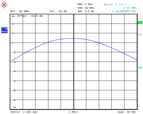
BLE 1Mbps_Low_Channel
