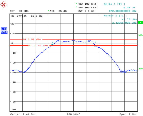
BLE 1Mbps_Middle_Channel
