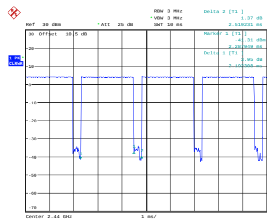
BLE 1Mbps_Middle_Channel
