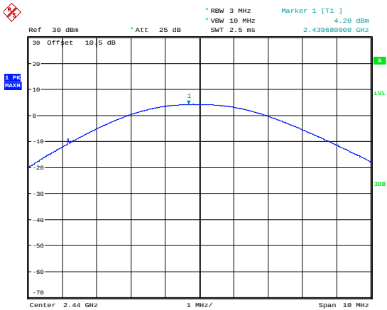
BLE 1Mbps_Middle_Channel
