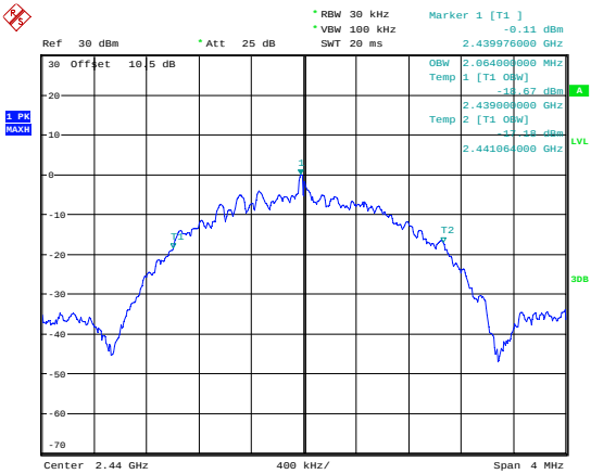
BLE 2Mbps_Middle_Channel
