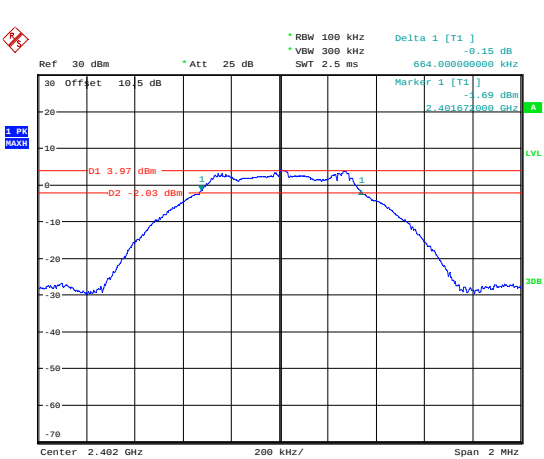
BLE 1Mbps_Low_Channel
