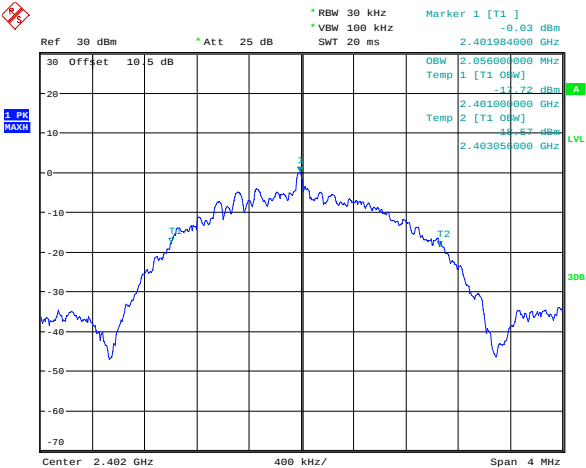
BLE 2Mbps_Low_Channel
