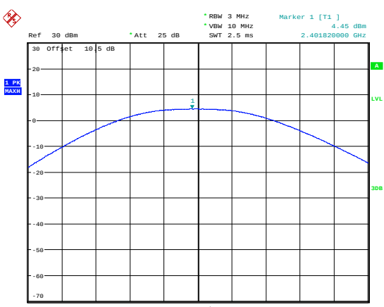
BLE 2Mbps_Low_Channel
