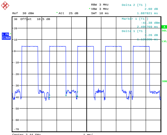
BLE 2Mbps_Middle_Channel
