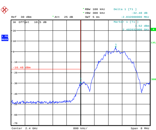
BLE 2Mbps_Low_Channel
