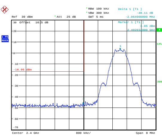
BLE 1Mbps_Low_Channel
