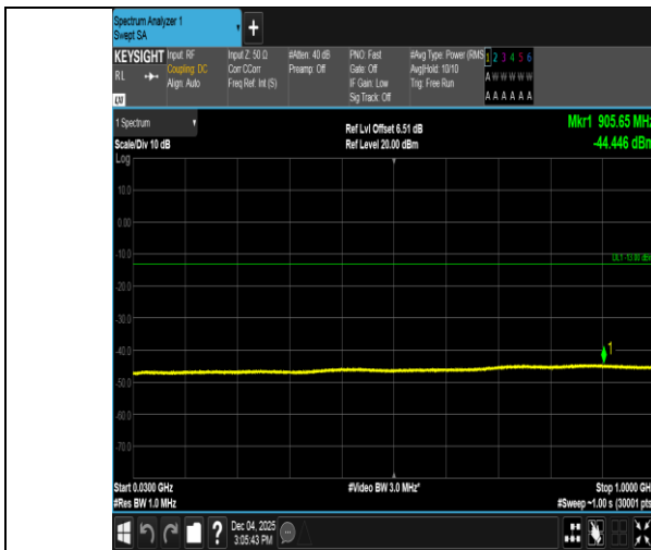
GSM1900-810-0-30~1000MHz-PASS
