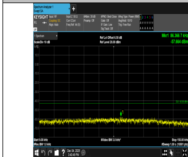
EGPRS1900-810-2-0.009~0.15MHz-PASS
