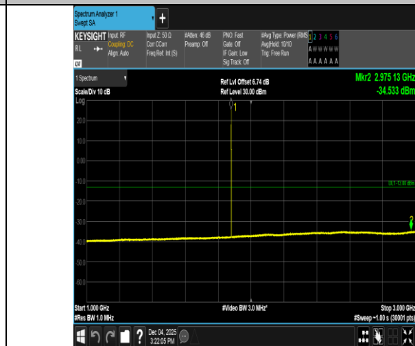
GPRS1900-661-0-1000~3000MHz-PASS
