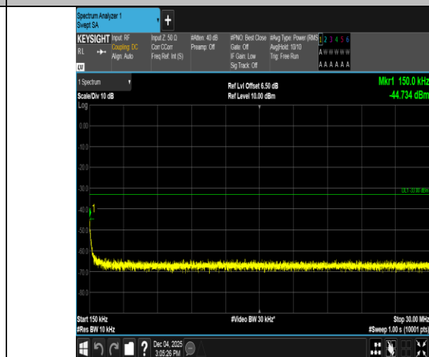
GSM1900-810-0-0.15~30MHz-PASS
