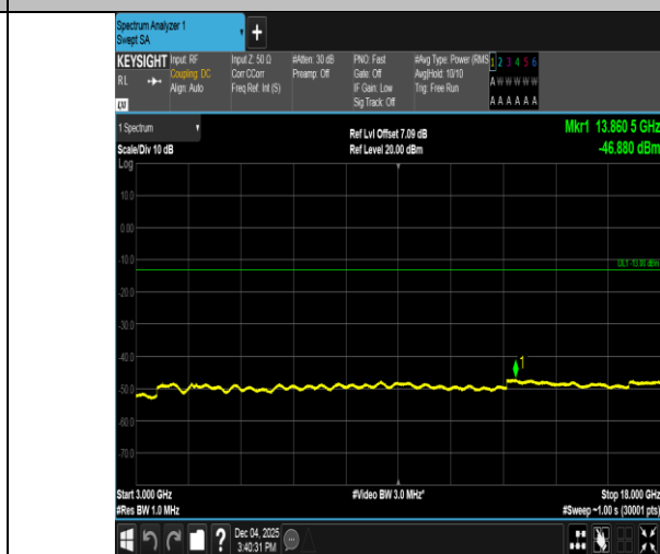
EGPRS1900-661-2-3000~18000MHz-PASS
