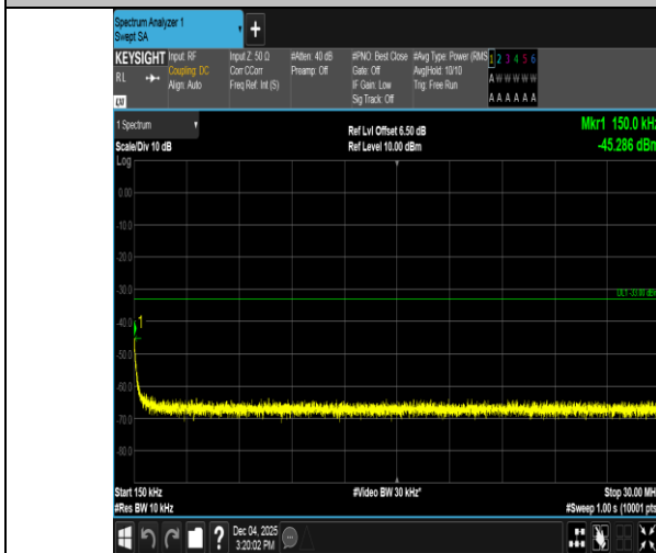
GPRS1900-512-0-0.15~30MHz-PASS
