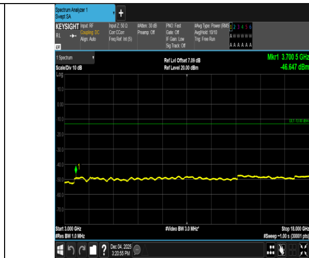
GPRS1900-512-0-3000~18000MHz-PASS
