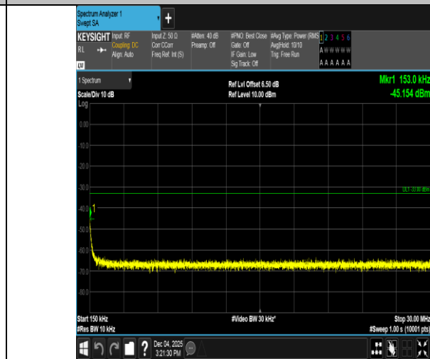
GPRS1900-661-0-0.15~30MHz-PASS
