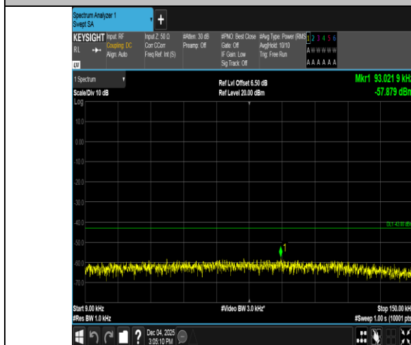
GSM1900-810-0-0.009~0.15MHz-PASS
