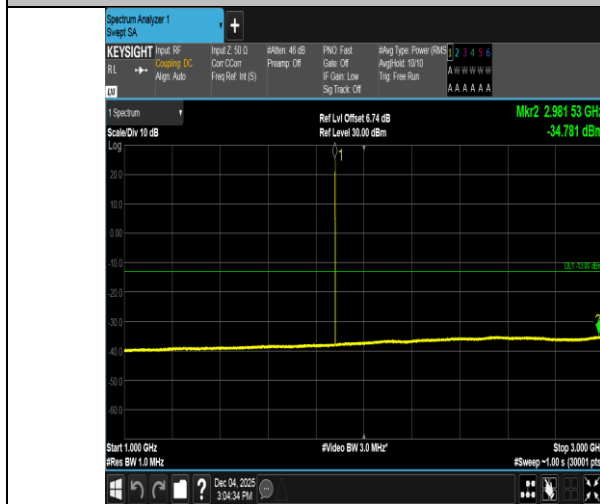
GSM1900-661-0-1000~3000MHz-PASS
