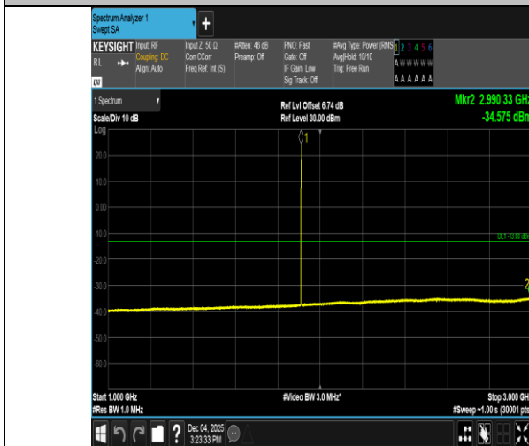
GPRS1900-810-0-1000~3000MHz-PASS
