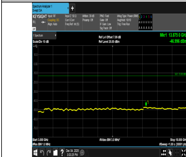
GSM1900-512-0-3000~18000MHz-PASS
