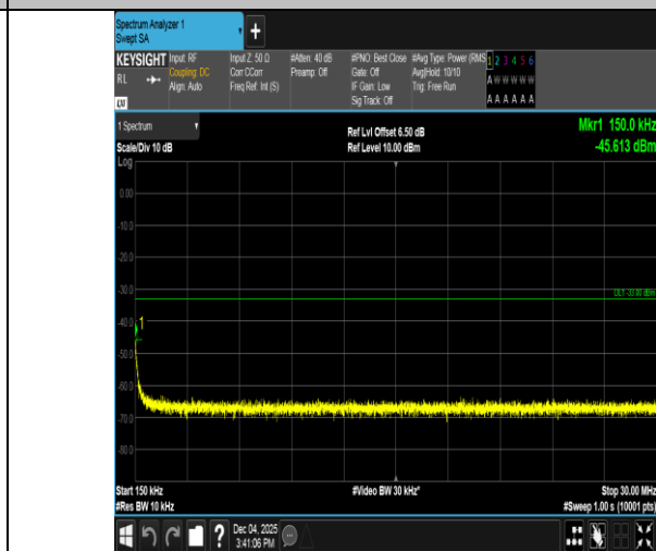
EGPRS1900-810-2-0.15~30MHz-PASS
