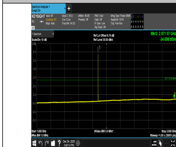
EGPRS1900-661-2-1000~3000MHz-PASS
