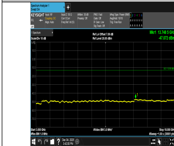
EGPRS1900-810-2-3000~18000MHz-PASS
