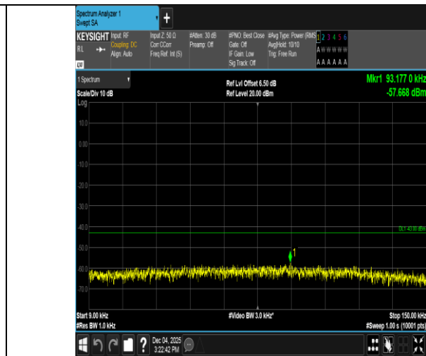
GPRS1900-810-0-0.009~0.15MHz-PASS
