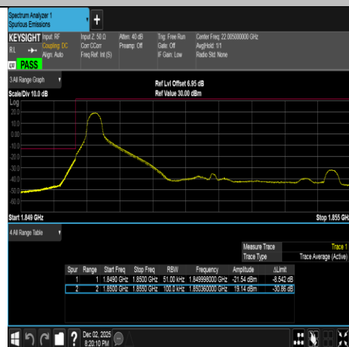
Band2-5MHz-16QAM-18625-1RB#0-PASS
