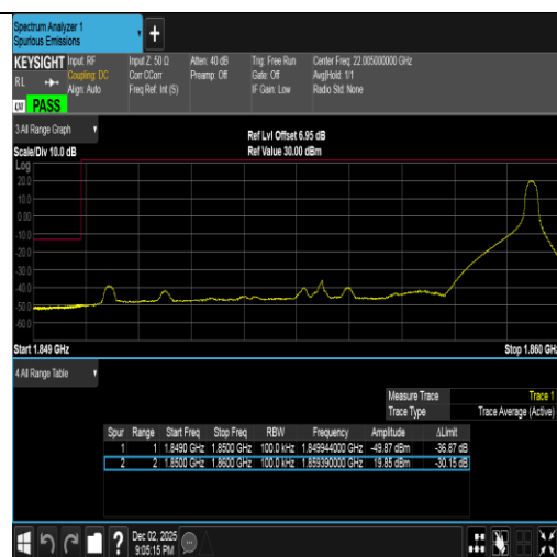
Band2-10MHz-QPSK-18650-1RB#49-PASS
