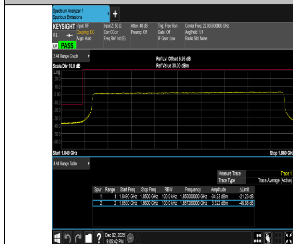
Band2-10MHz-QPSK-18650-50RB#0-PASS
