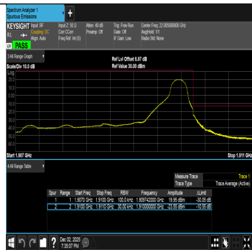
Band2-3MHz-QPSK-19185-1RB#14-PASS
