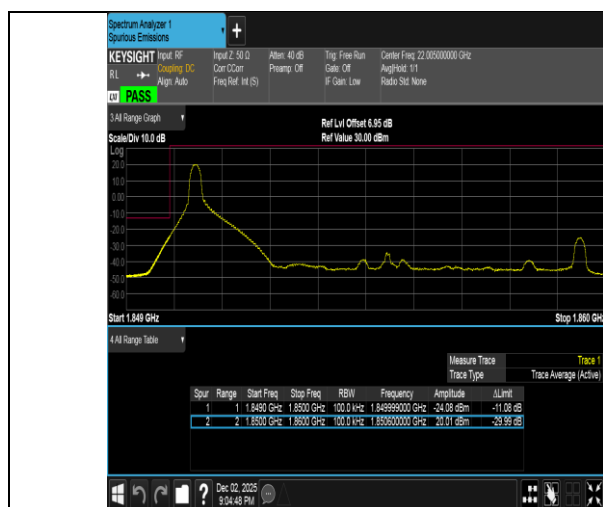
Band2-10MHz-QPSK-18650-1RB#0-PASS
