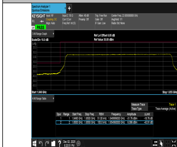
Band2-5MHz-QPSK-18625-25RB#0-PASS
