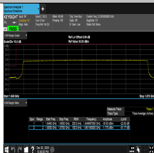
Band2-20MHz-16QAM-18700-100RB#0-PASS
