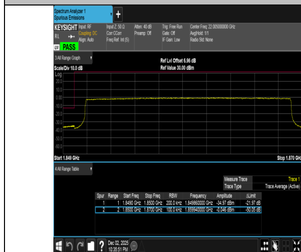
Band2-20MHz-QPSK-18700-100RB#0-PASS
