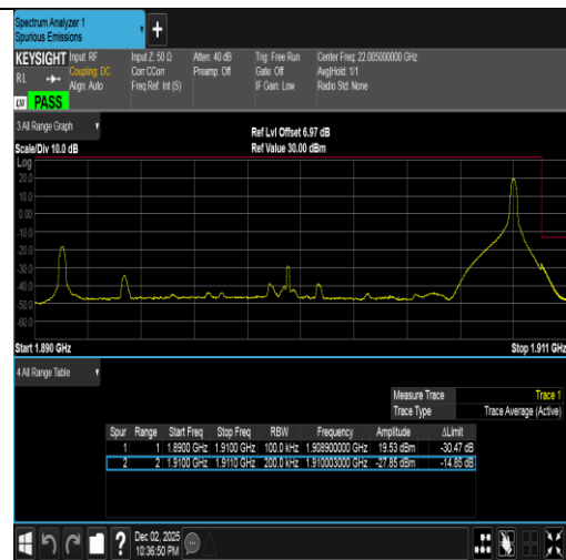
Band2-20MHz-QPSK-19100-1RB#99-PASS
