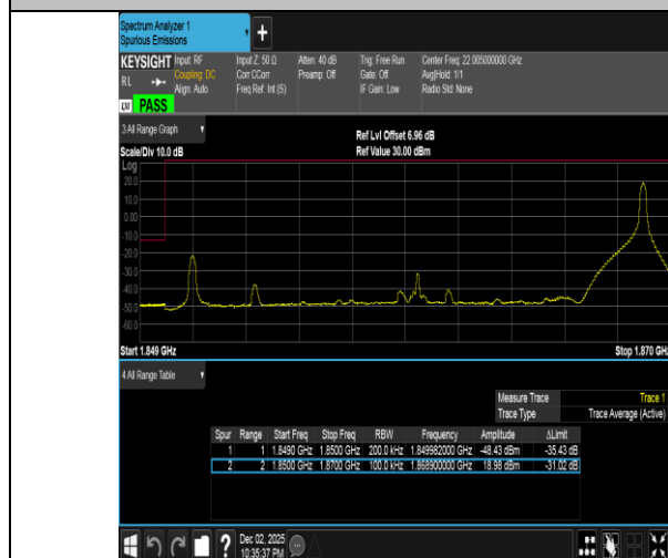
Band2-20MHz-16QAM-18700-1RB#99-PASS
