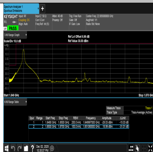
Band2-20MHz-16QAM-18700-1RB#0-PASS
