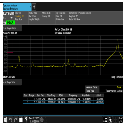
Band2-20MHz-QPSK-18700-1RB#99-PASS
