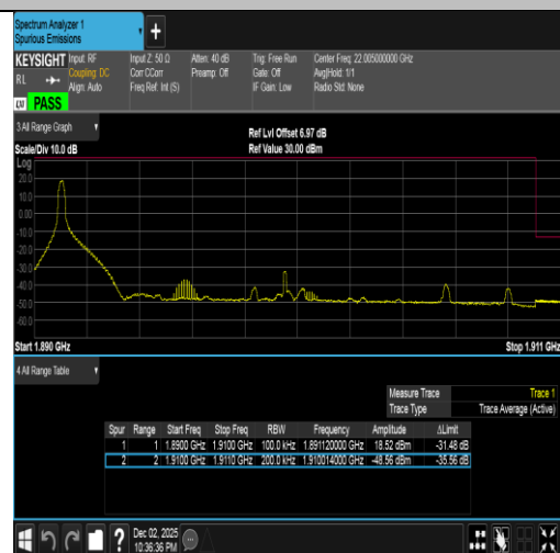
Band2-20MHz-16QAM-19100-1RB#0-PASS
