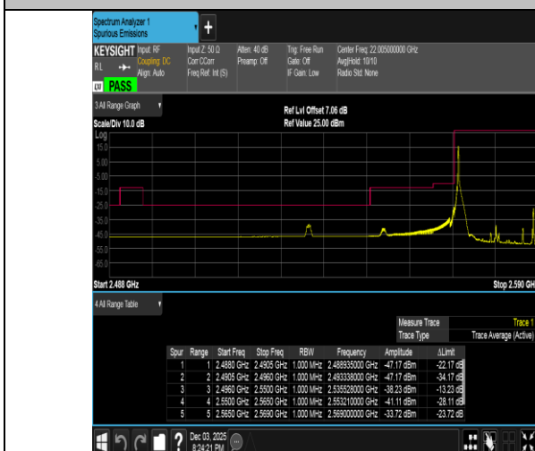
Band38-20MHz-QPSK-37850-1RB#0-PASS
