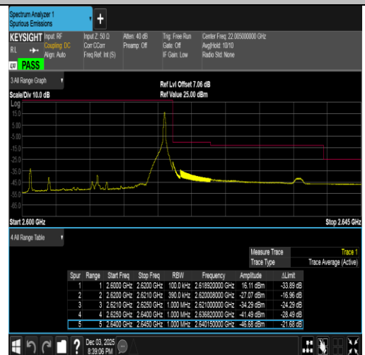
Band38-20MHz-QPSK-38150-1RB#99-PASS
