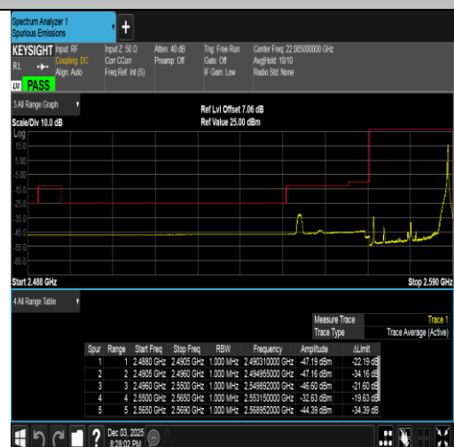
Band38-20MHz-QPSK-37850-1RB#99-PASS
