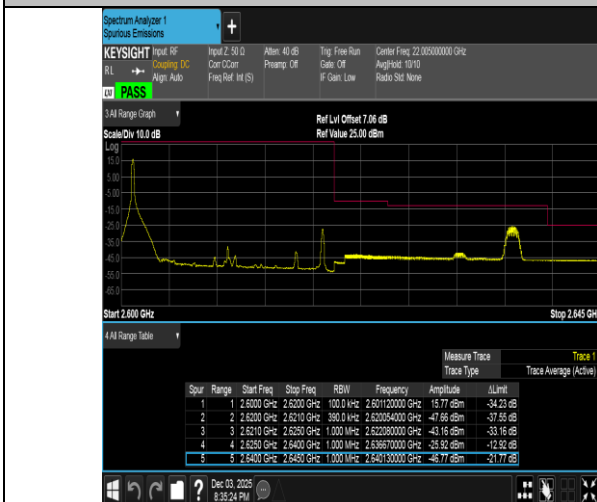
Band38-20MHz-QPSK-38150-1RB#0-PASS
