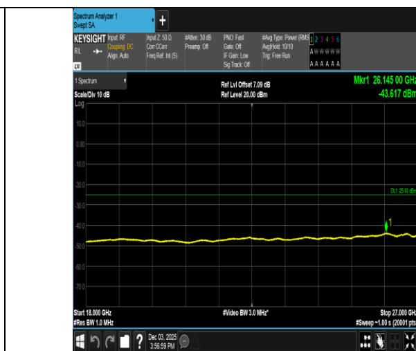
Band38-5MHz-QPSK-38000-25RB#0-18000~27000-PASS
