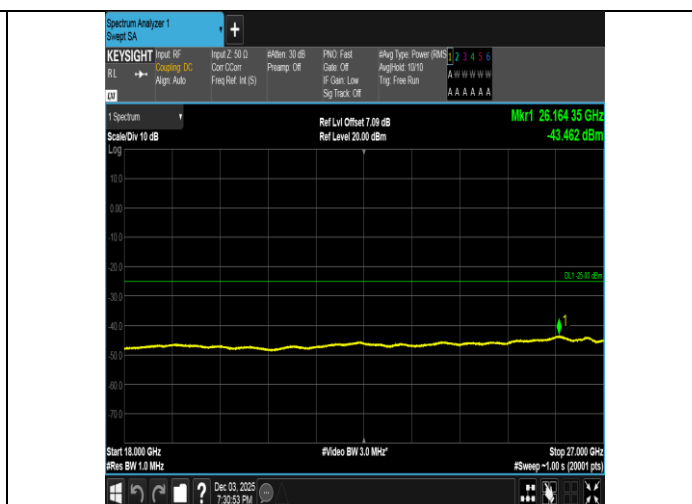
Band38-15MHz-16QAM-38000-1RB#0-18000~27000-PASS
