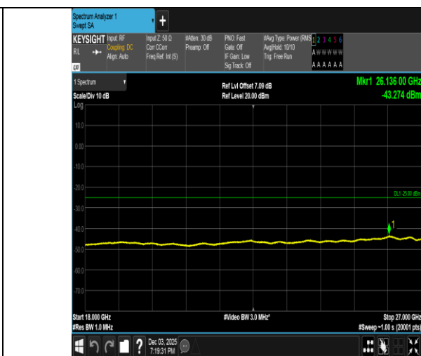
Band38-15MHz-QPSK-37825-1RB#74-18000~27000-PASS
