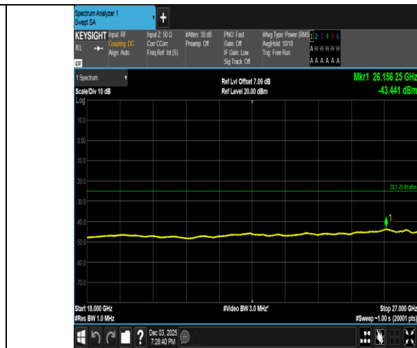
Band38-15MHz-QPSK-38000-1RB#0-18000~27000-PASS
