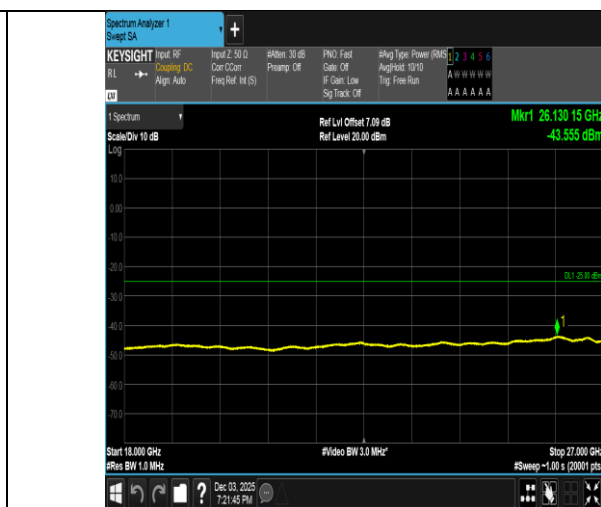
Band38-15MHz-16QAM-37825-1RB#74-18000~27000-PASS
