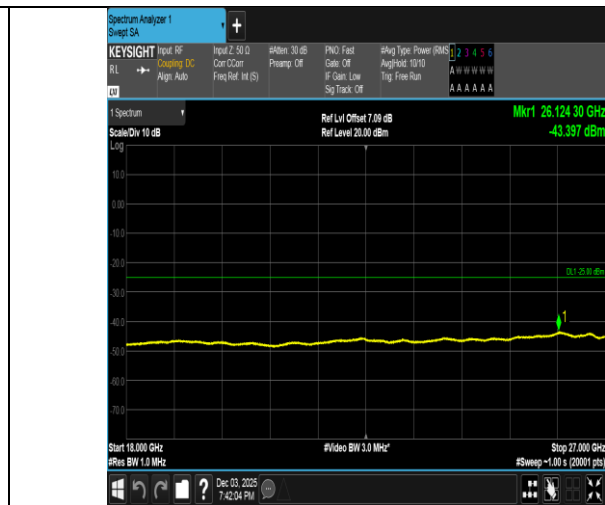
Band38-15MHz-QPSK-38175-1RB#0-18000~27000-PASS
