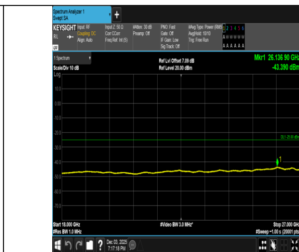
Band38-15MHz-16QAM-37825-1RB#0-18000~27000-PASS
