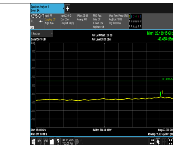
Band38-15MHz-QPSK-38000-1RB#74-18000~27000-PASS
