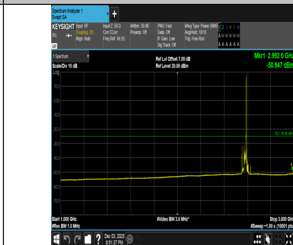
Band38-20MHz-QPSK-37850-1RB#99-1000~3000-PASS
