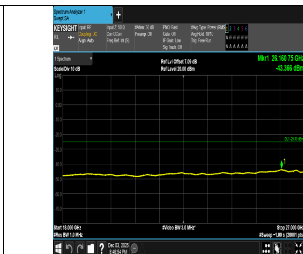
Band38-20MHz-QPSK-37850-1RB#0-18000~27000-PASS
