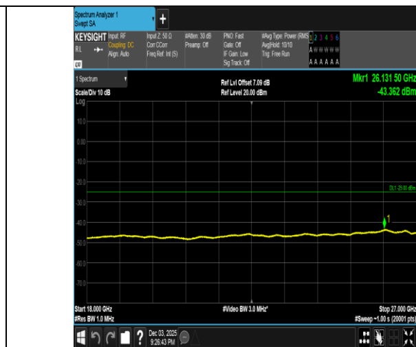
Band38-20MHz-QPSK-38000-1RB#99-18000~27000-PASS
