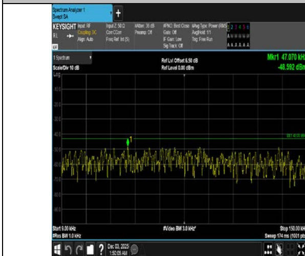
Band4-10MHz-QPSK-20000-50RB#0-0.009~0.15-PASS
