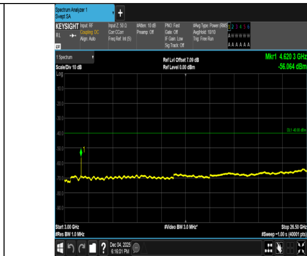
Band40(2305-2315)-10MHz-QPSK-38750-50RB#0-3000~26500-PASS
