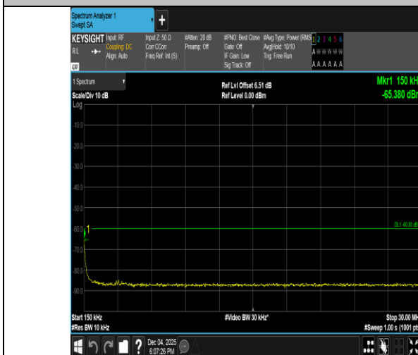
Band40(2305-2315)-10MHz-QPSK-38750-1RB#0-0.15~30-PASS
