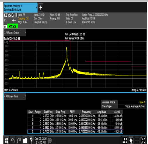
Band41-20MHz-QPSK-41490-1RB#99-PASS
