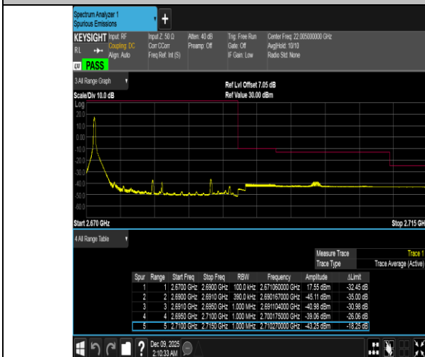
Band41-20MHz-QPSK-41490-1RB#0-PASS
