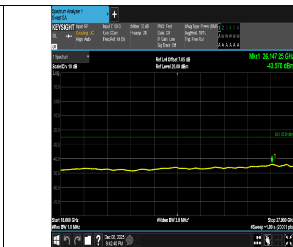
Band41-5MHz-QPSK-40620-25RB#0-18000~27000-PASS
