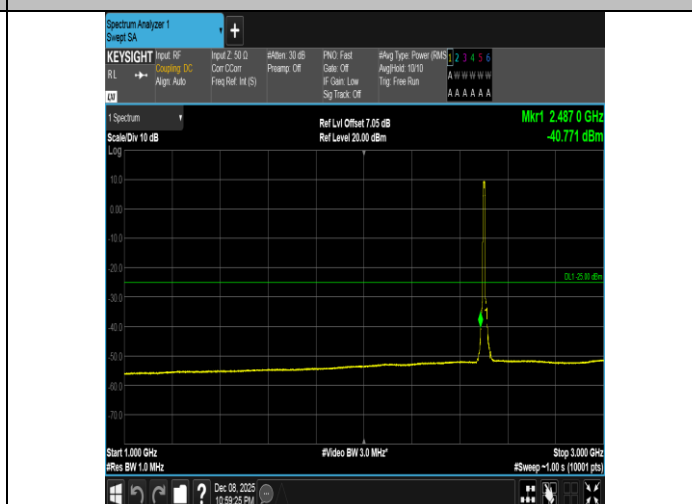
Band41-10MHz-QPSK-39700-50RB#0-1000~3000-PASS
