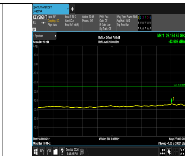
Band41-5MHz-16QAM-41565-1RB#0-18000~27000-PASS
