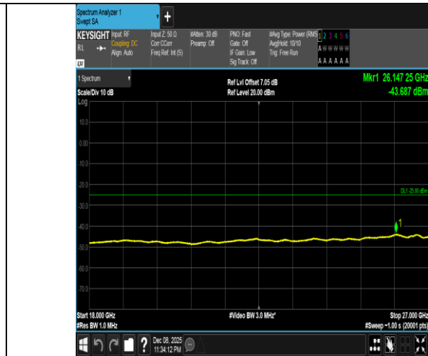
Band41-10MHz-QPSK-41540-50RB#0-18000~27000-PASS
