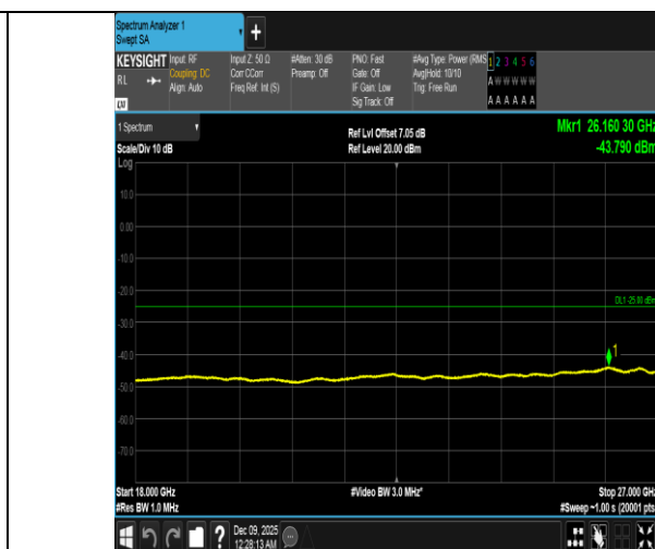
Band41-15MHz-QPSK-39725-1RB#0-18000~27000-PASS
