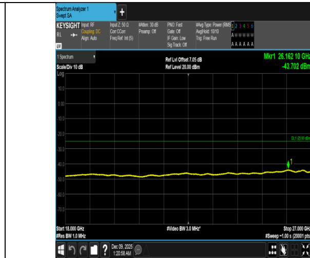
Band41-15MHz-16QAM-41515-1RB#74-18000~27000-PASS
