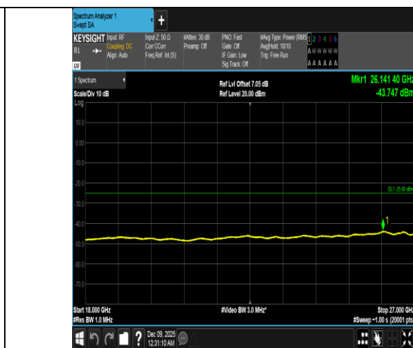
Band41-15MHz-16QAM-39725-1RB#0-18000~27000-PASS
